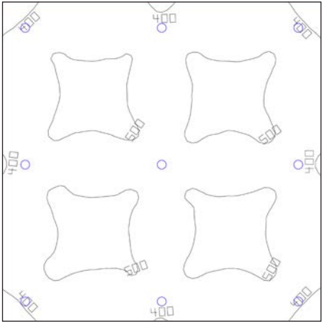
2018.190 燈具配置參考 燈具間距 2.5x2.5m 安裝高度 3.5m
