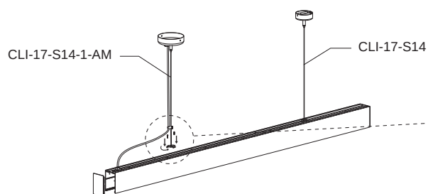
用於吊掛形式的固定安裝
