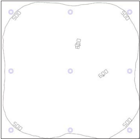
2018.475 燈具配置參考 燈具間距 2.5x2.5m 安裝高度 3.5m
