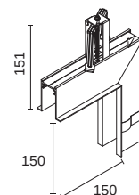
SDF-04 有邊框軌道-7型
