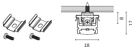
NS-0589 固定夾 (選配)
