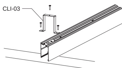
使用懸掛夾的固定形式
